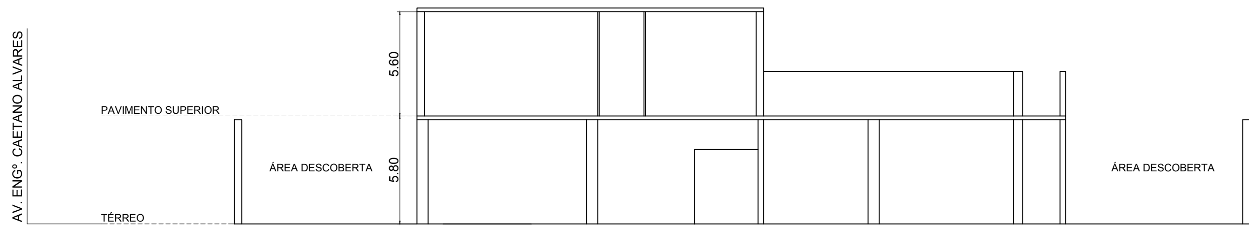
CORTE A-A
